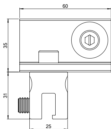
Falzklemme RD-80 BW Uni
