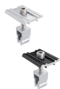
middle 36-42 clamp uni ic 50 / mittelklemme 36-42 uni ik 50 material: EN AW-6063 T66 / A2-70
