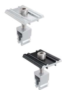
middle 30-35 clamp uni ic 50 / mittelklemme 30-35 uni ik 50 material: EN AW-6063 T66 / A2-70
