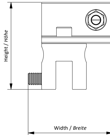
winkelstehfalzklemme bw uni angled seam clamp bw uni
