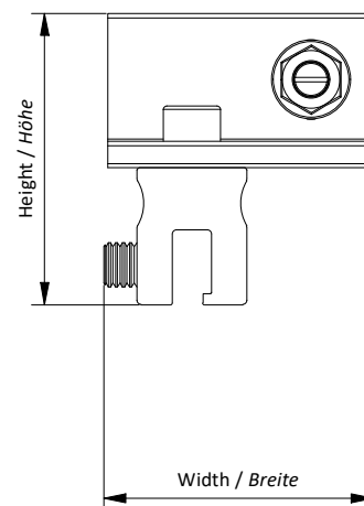
doppelstehfalzklemme bw uni double seam clamp bw uni
