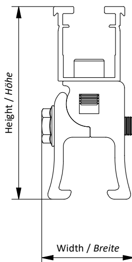
falzklemme k15 bk uni seam clamp k15 bk uni
