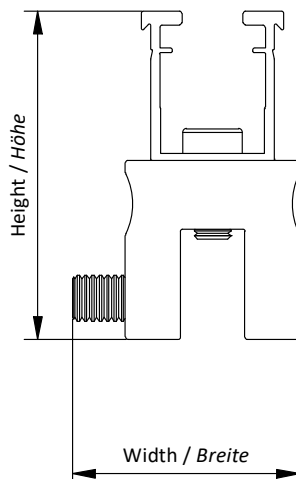
winkelstehfalzklemme bk uni angled seam clamp bk uni
