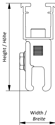
falzklemme rd-80 bk uni seam clamp rd-80 bk uni
